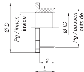
Dimensions Design A knurled Dimensionen Bauform A randriert
