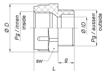
Dimensions Design B hexagonal Dimensionen Bauform B sechskant
